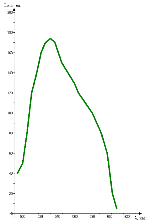
Fig. 2. Spectrul fotoluminescenței nanoparticulelor CdS în matrița polimerică a SEVILENului.
