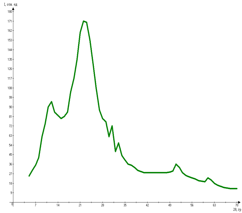
Fig. 1. Spectrul de difracție de raze X al nanoparticulelor CdS în matrița polimerică a SEVILENului.
